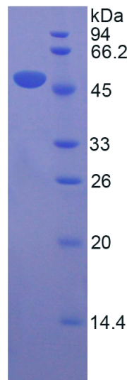
15% SDS-PAGE
