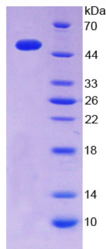
15% SDS-PAGE
