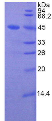
15% SDS-PAGE
