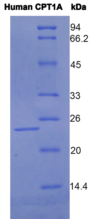
15% SDS-PAGE
